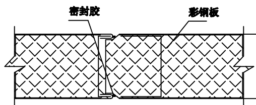
企口式嵌入式节点
