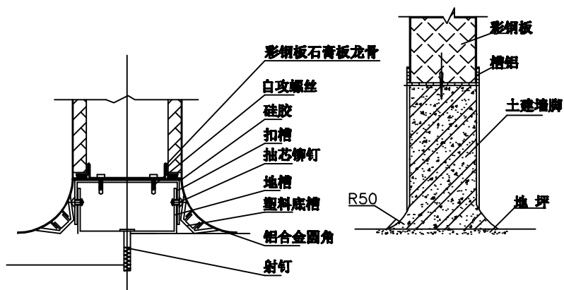
彩钢板与地槽连接形式
