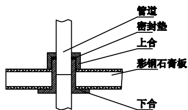
管道穿越吊顶密封形式
