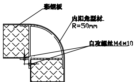
包柱内阳角作法
