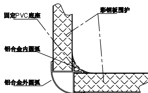
企口式嵌入式节点
